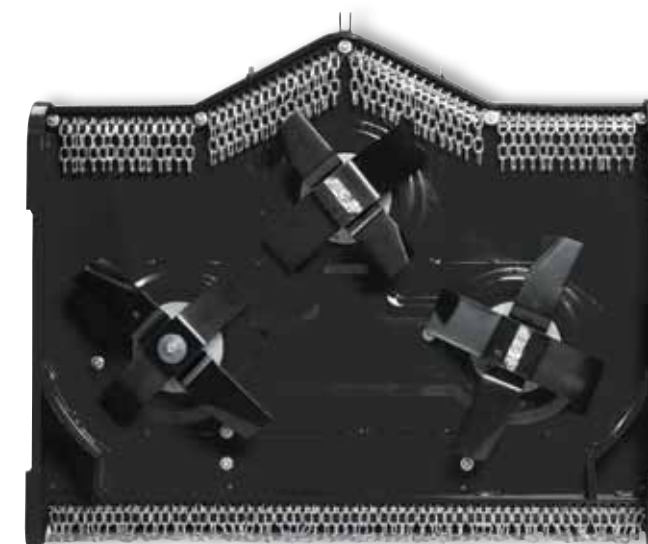
Het Hoog Gras Mulchdek is voorzien van 6 messen (2 per as). Doordat er gebruik gemaakt wordt van 3 lagerpotten is de kans op schade, bij het raken van een stronk of grote steen, aanzienlijk kleiner dan bij een maaidek met maar 1 lagerpot. Niet de goedkoopste oplossing maar wel de beste.
